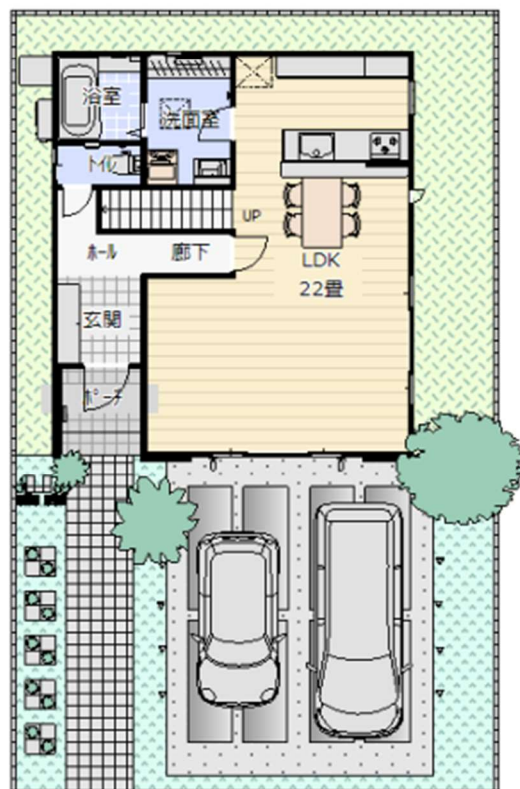
1階平面図
