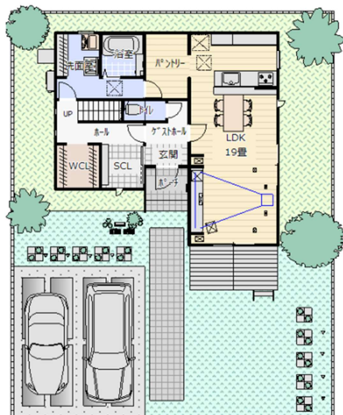
1 階平面図
