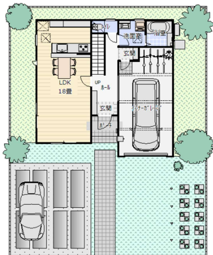
1階平面図
