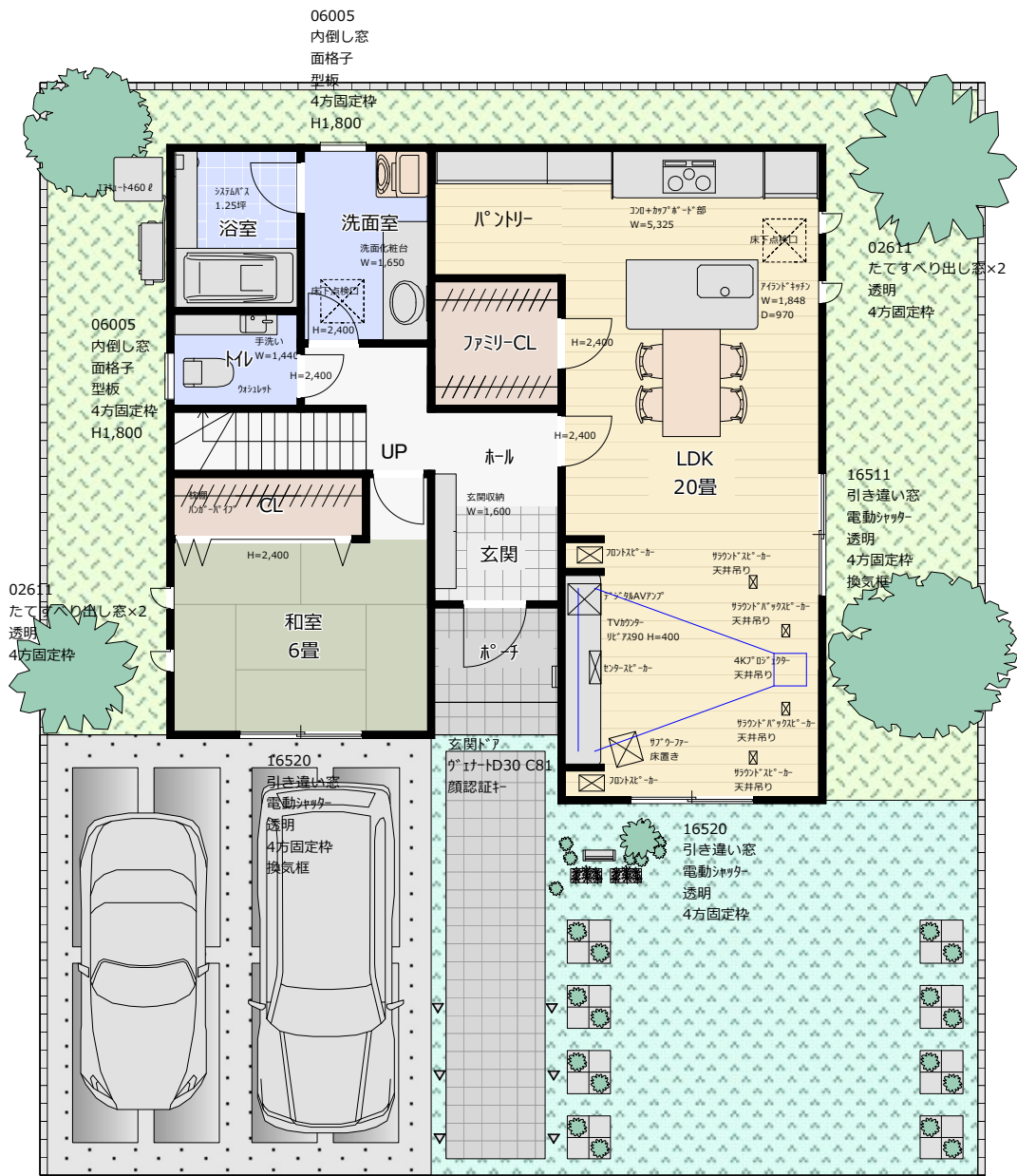
1 階平面図
